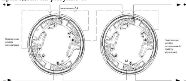
Рисунок 1 – Схема подключения извещателя пожарного теплового максимального адресного ИП-101-1-A2 (HNAR-360).
