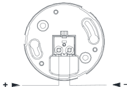
Рисунок 3 – Схема подключения выносного устройства индикации RI – 681
