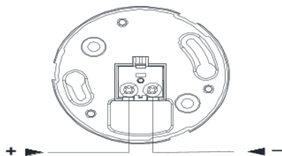
Рисунок 3 – Схема подключения выносного индикатора RI – 681
