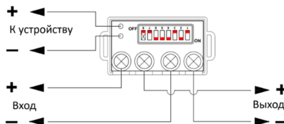
Рисунок 1 – Схема подключения модуля вывода
